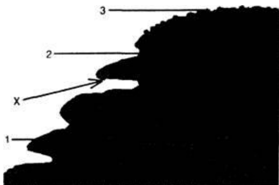
Рис. 4.2. Стратиграфия места находки у подножия Монте-Редонду, в районе Отта (Португалия), где Дж. Беллуччи нашел кремневое орудие:
